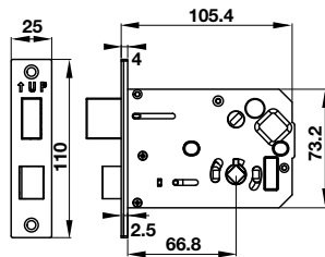
Thân khóa nhỏ Small mortise
